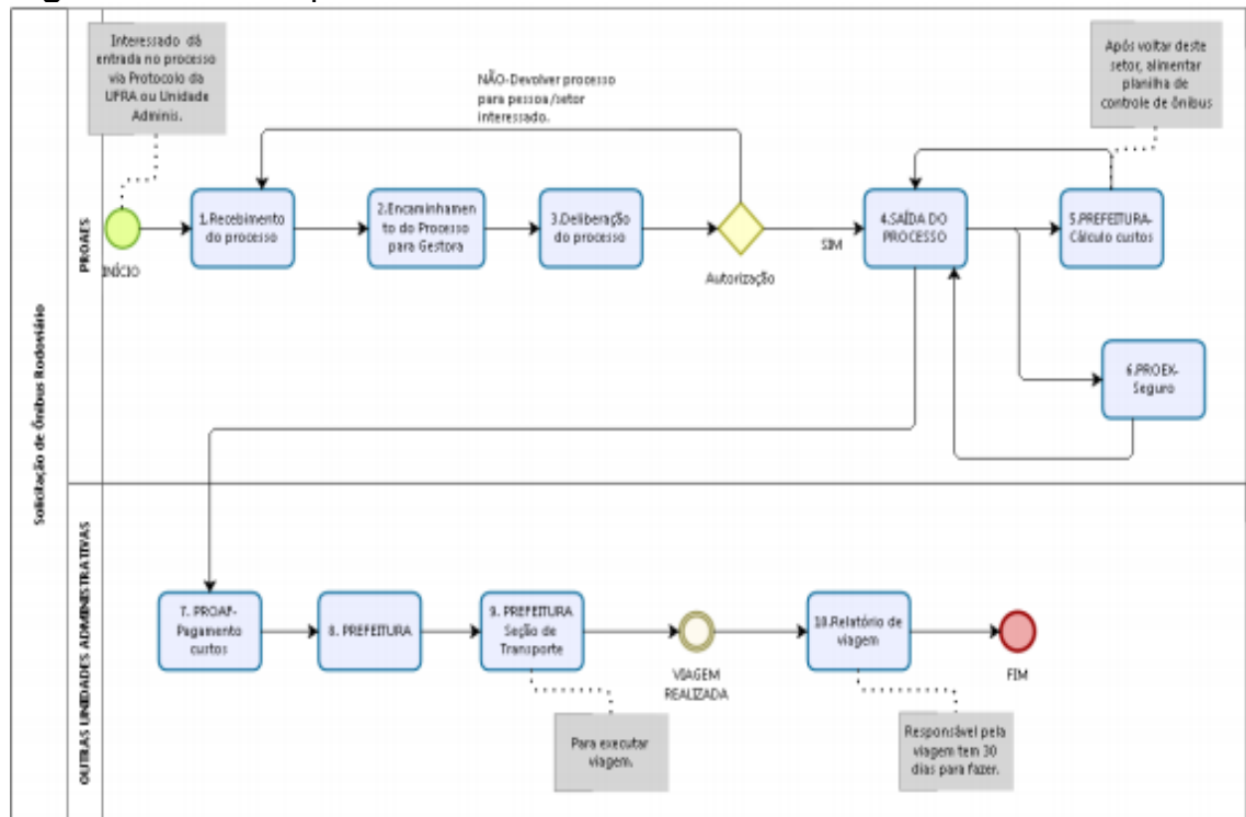
Figura 2: Fluxo de processo do Edital de ônibus rodoviário
